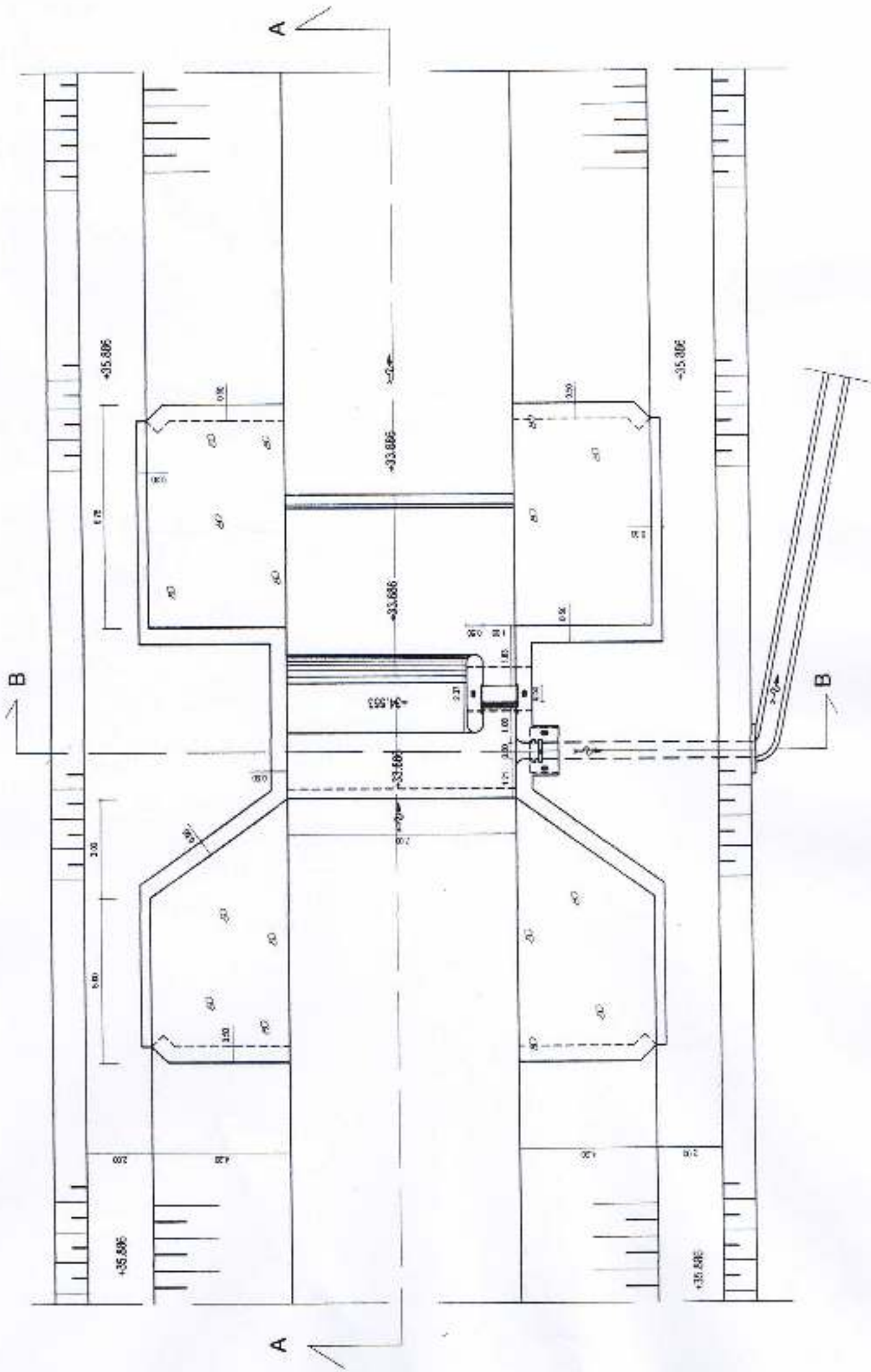
Denah Bendung Sungai Bojong SKALA 1:1000
